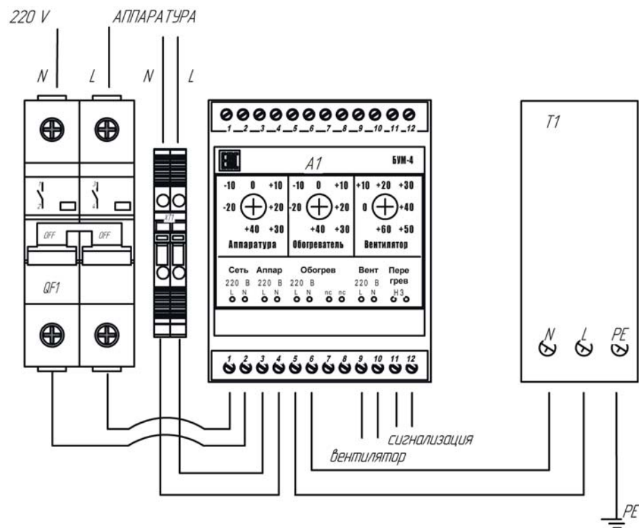
Рис. 2. Схема расключения. Фрагмент
