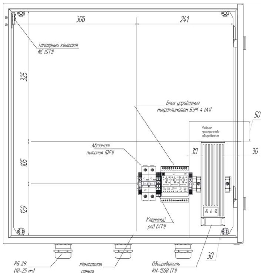
Рис. 1. Внешний вид с открытой дверью, 90 °
